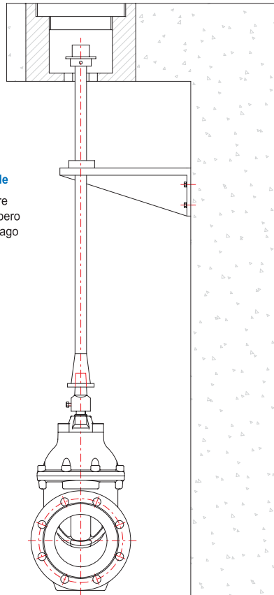
Valve box Boîte vanne Scatola valvola Caja de Válvula
